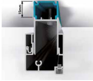
Profilé d'éclaircissement 508838
